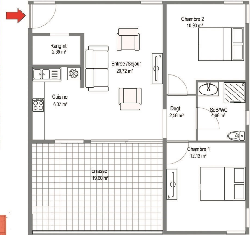
NIVEAU RdC
