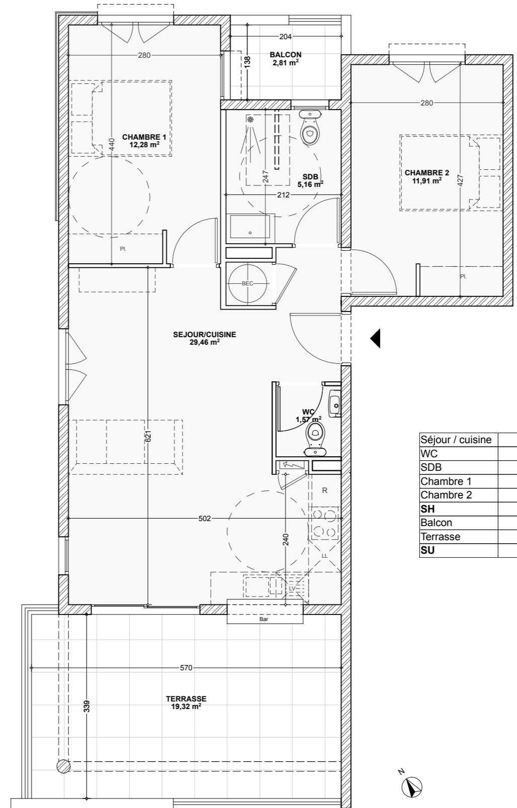
PLAN APPARTEMENT
