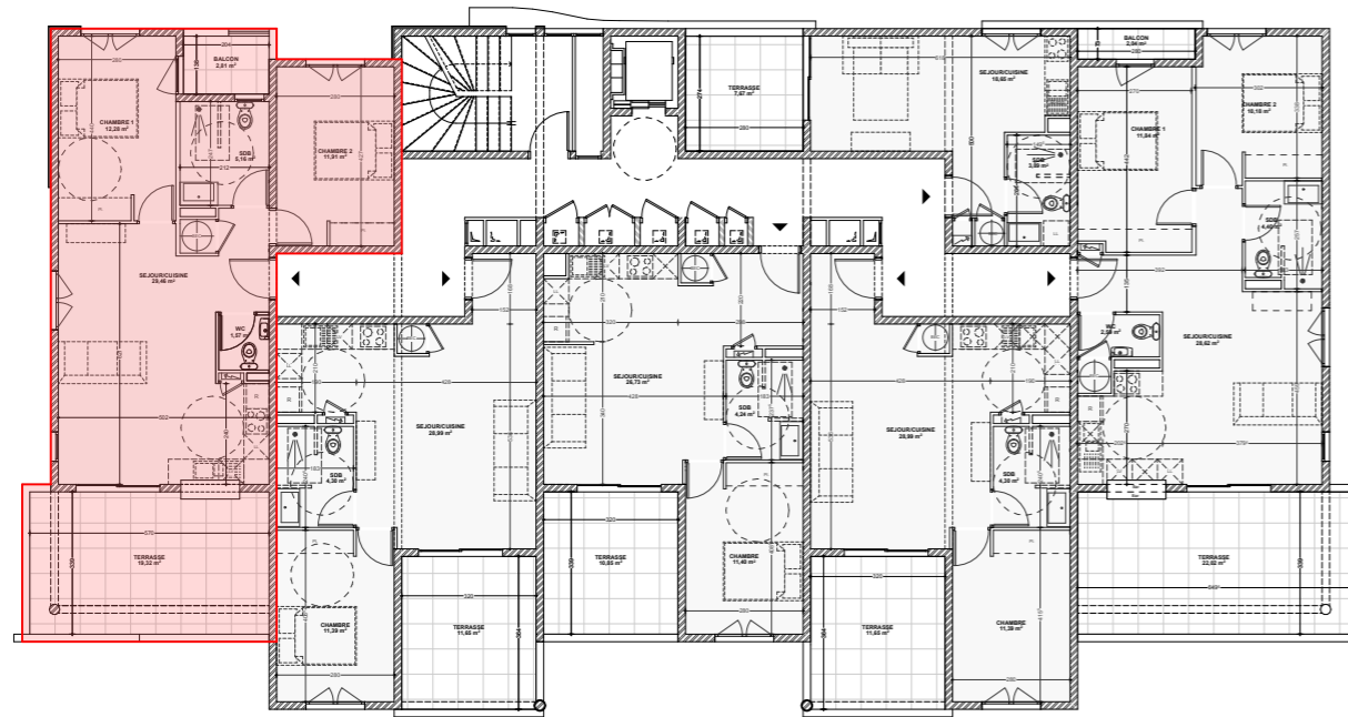
PLAN NIVEAU
