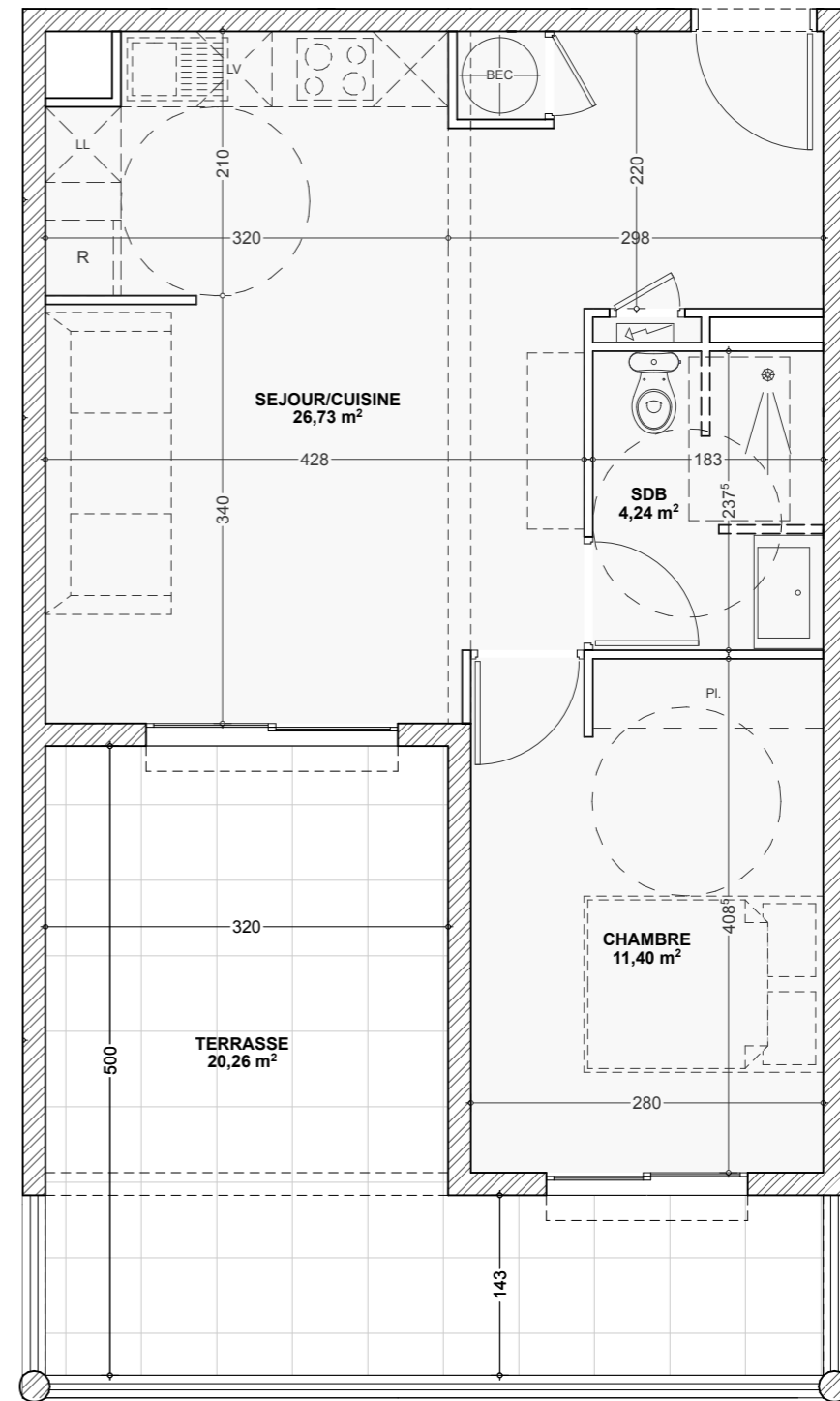
PLAN APPARTEMENT
