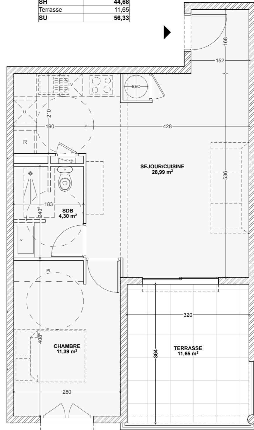
PLAN APPARTEMENT
