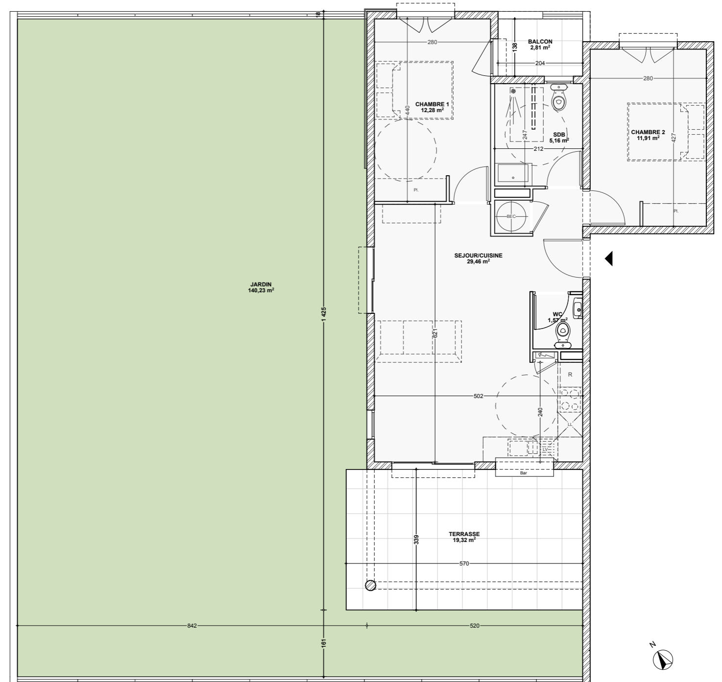
PLAN APPARTEMENT
