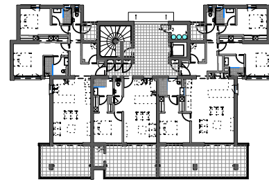
Niveau R+7 (Logements)
