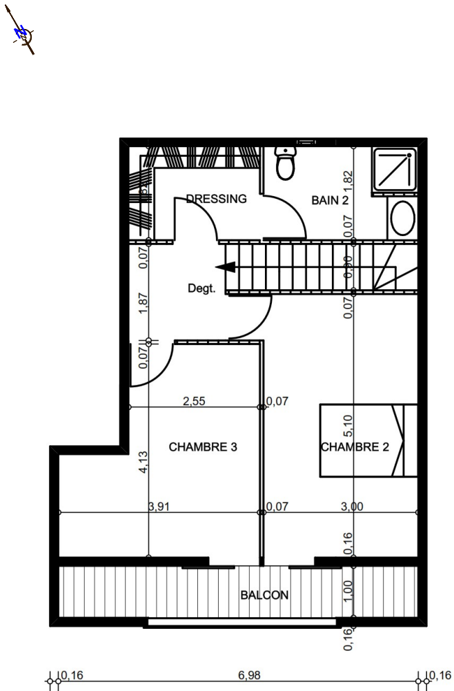
T4 COMBLES
