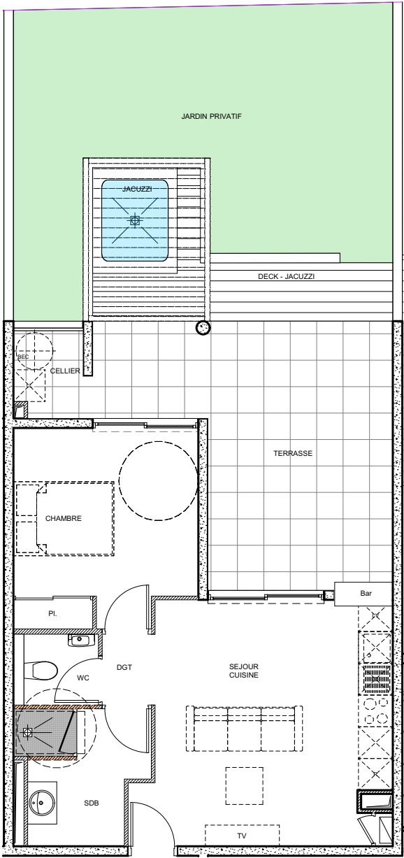
PLAN APPARTEMENT
