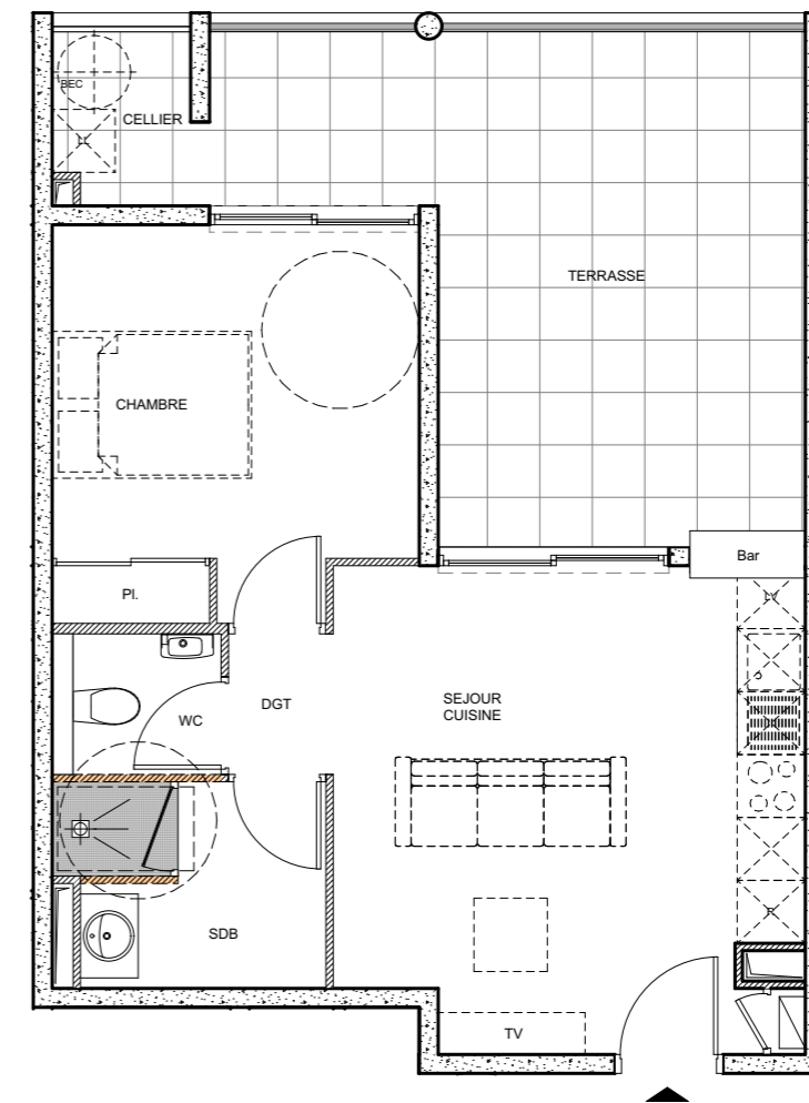
PLAN APPARTEMENT
