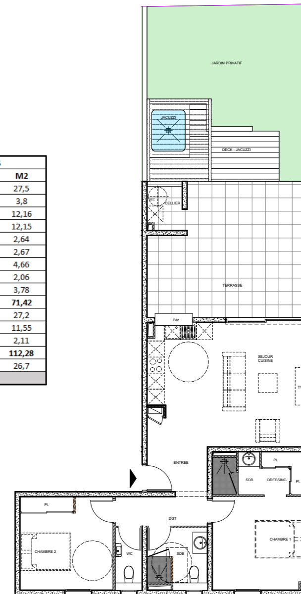
PLAN APPARTEMENT
