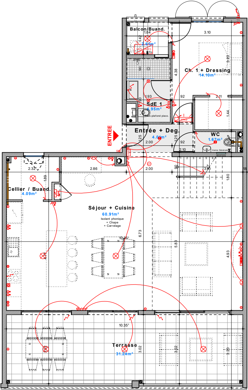
Logement (R+6)
