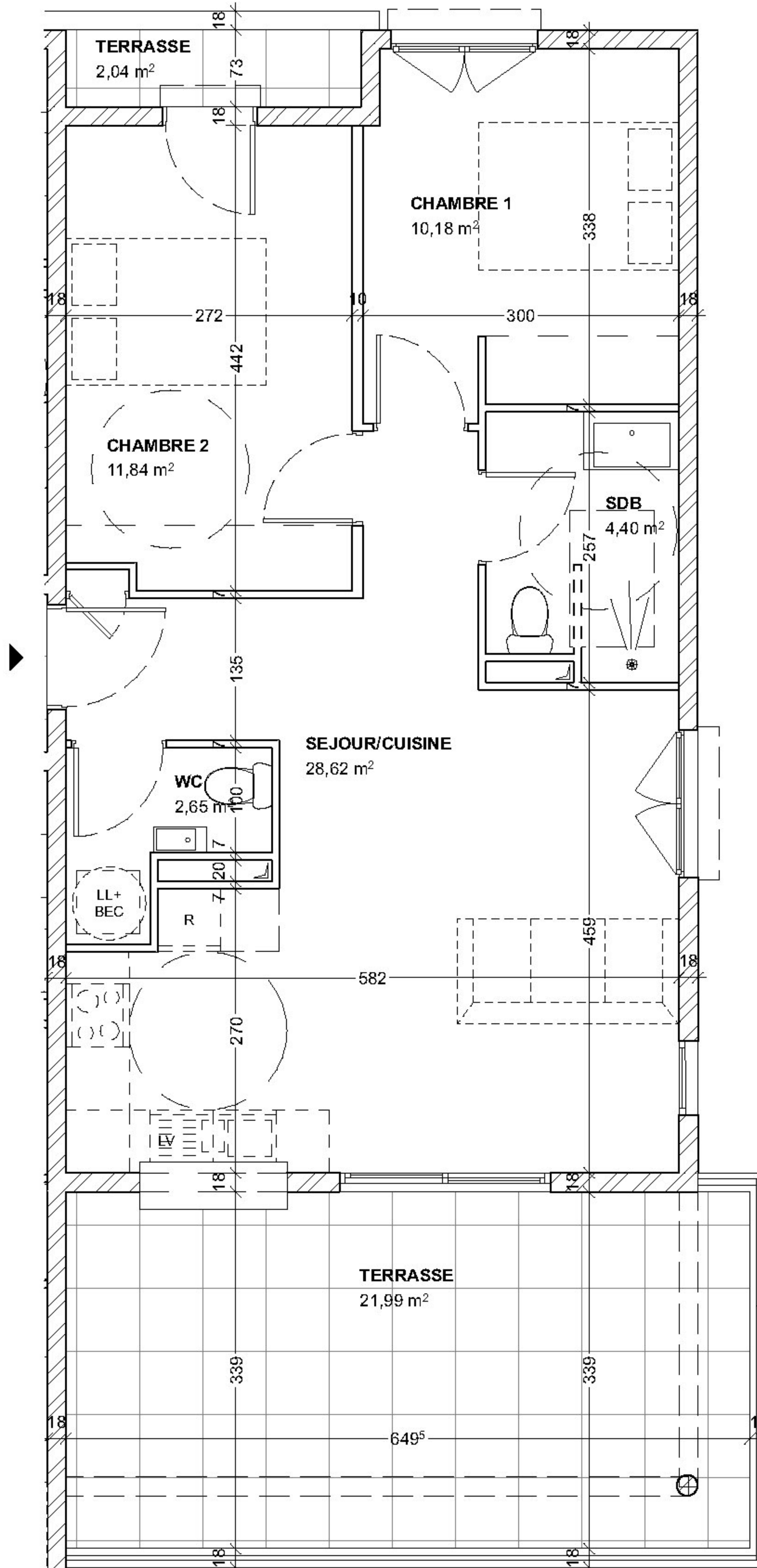
PLAN APPARTEMENT
