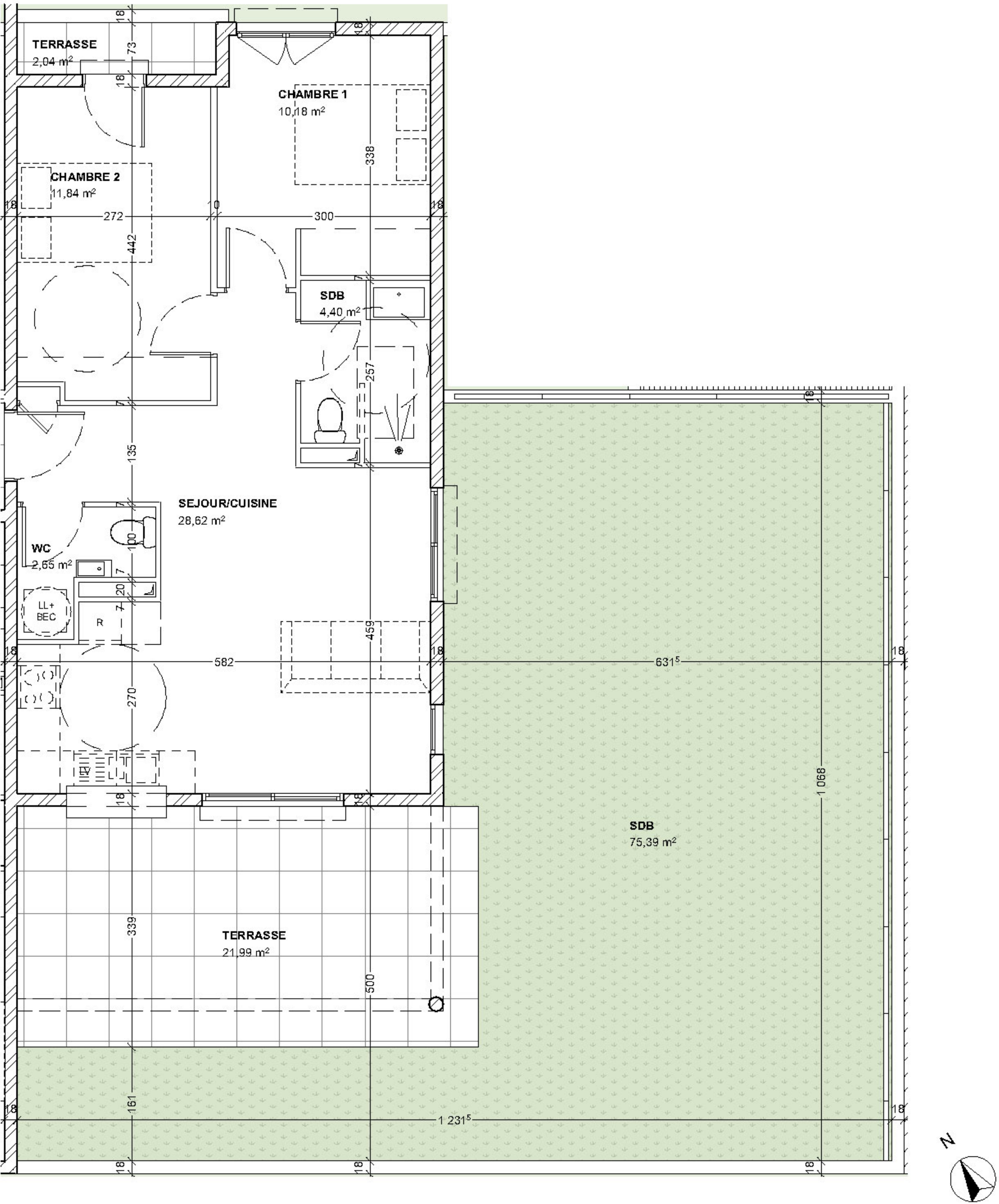
PLAN APPARTEMENT
