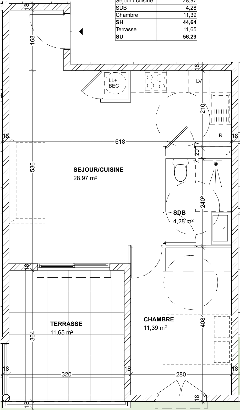
PLAN APPARTEMENT
