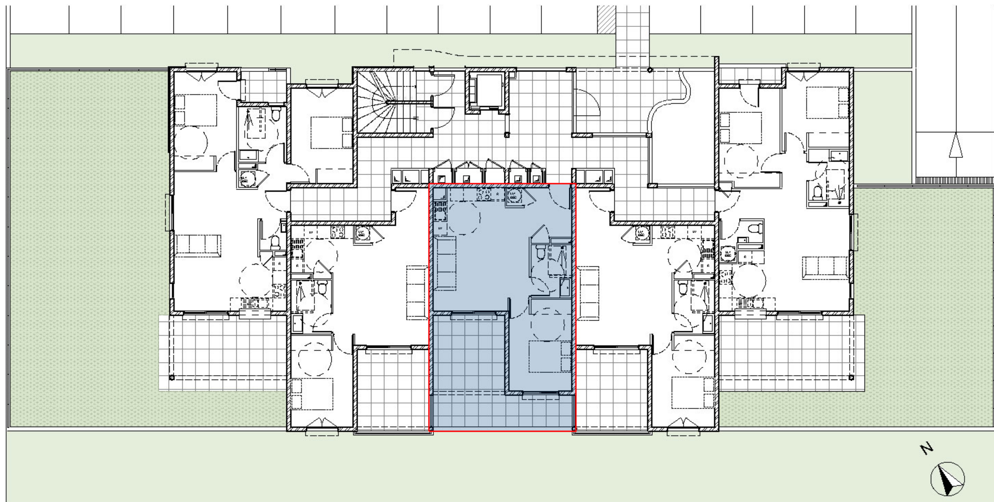
PLAN NIVEAU
