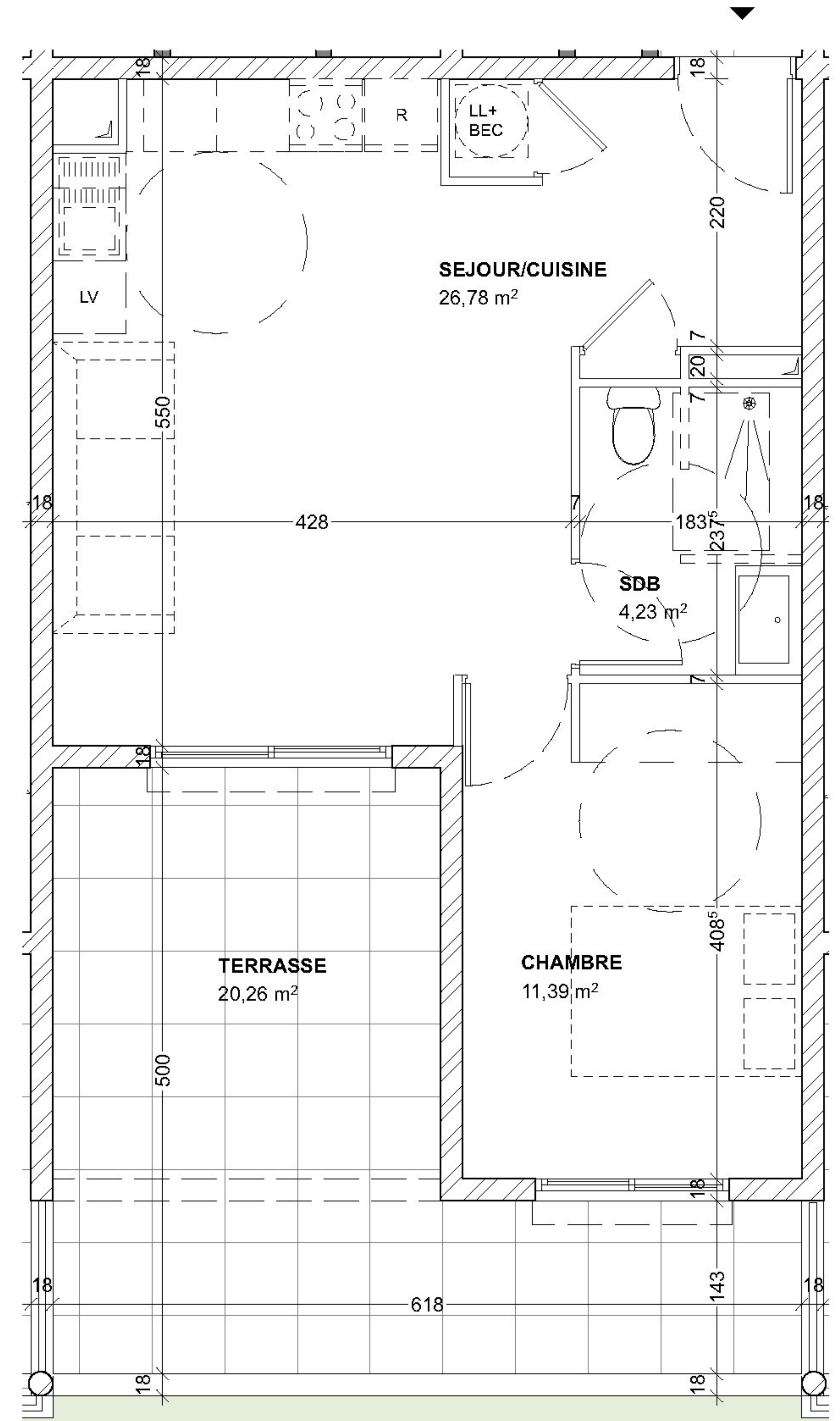
PLAN APPARTEMENT
