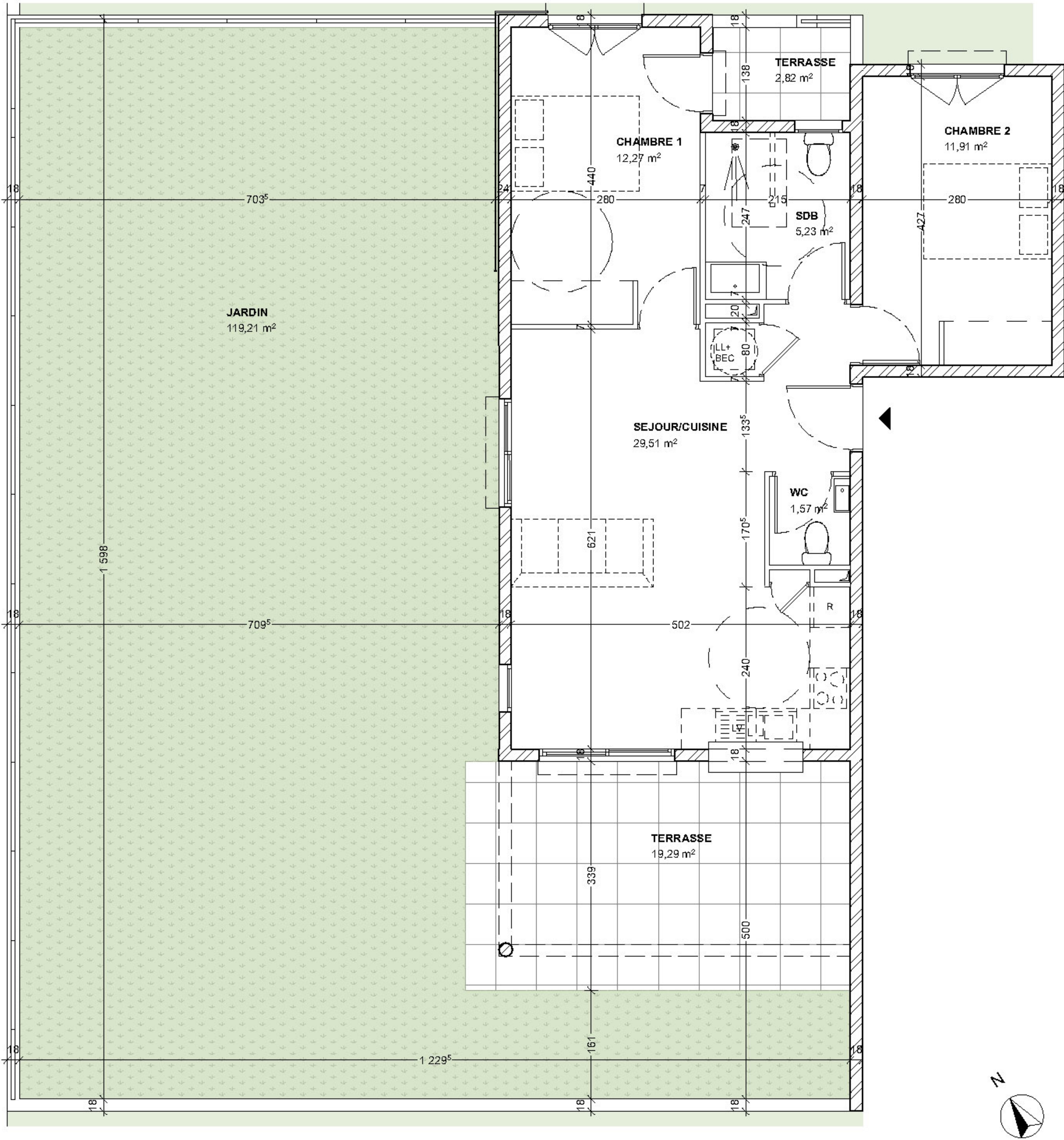
PLAN APPARTEMENT
