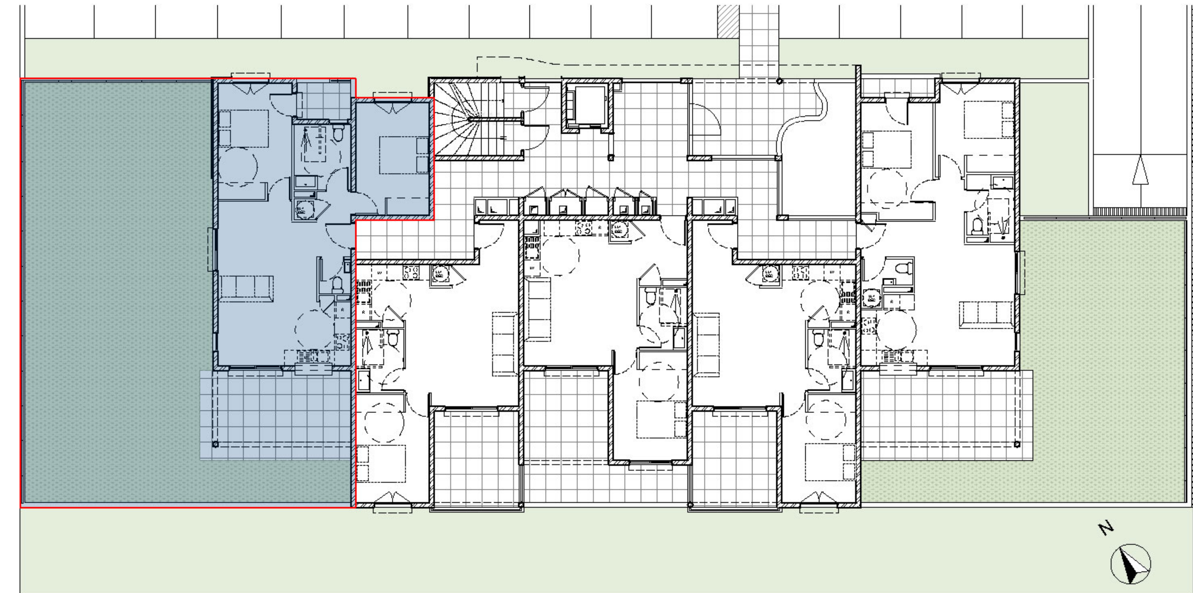
PLAN NIVEAU
